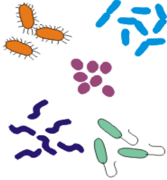
سند3:الكائنات المحللة
