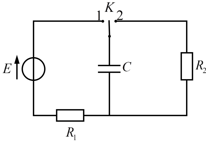
الشكل 4. دائرة تجربة شحن وتفريغ مكثفة
