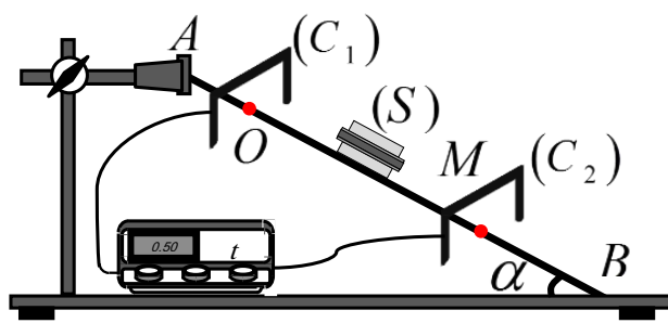
الشكل 9. حركة جسم صلب فوق مستوي مائل
