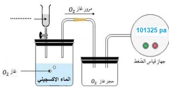
البروتوكول التجريبي لقياس ضغط غاز
