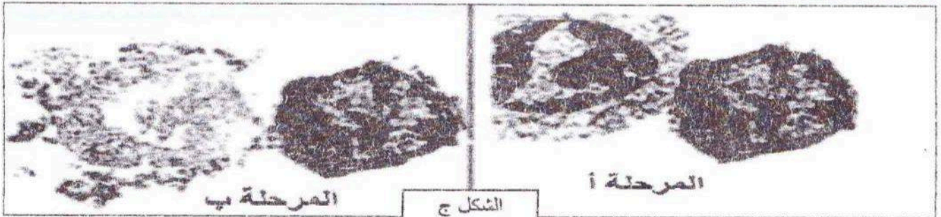
الشكل (ب) : جدول الترميزات و ما يقابلها من أحماض أمينية
