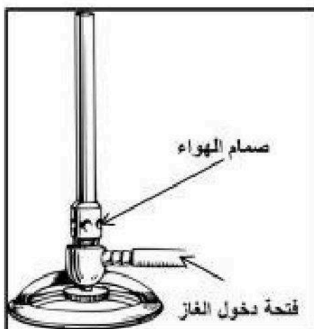
موقد بنزن
